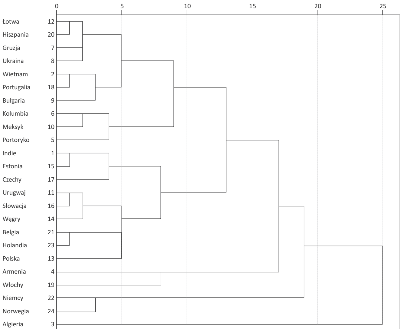
Rysunek 1. Dendrogram* z wykorzystaniem średniego powiązania (między grupami). Łączone skupienia (odległości przeskalowane).
